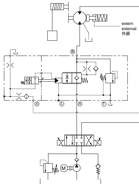
Schaltbeispiel für SVT (B → T) für Wegeventile mit geschlossener Mittelstellung
